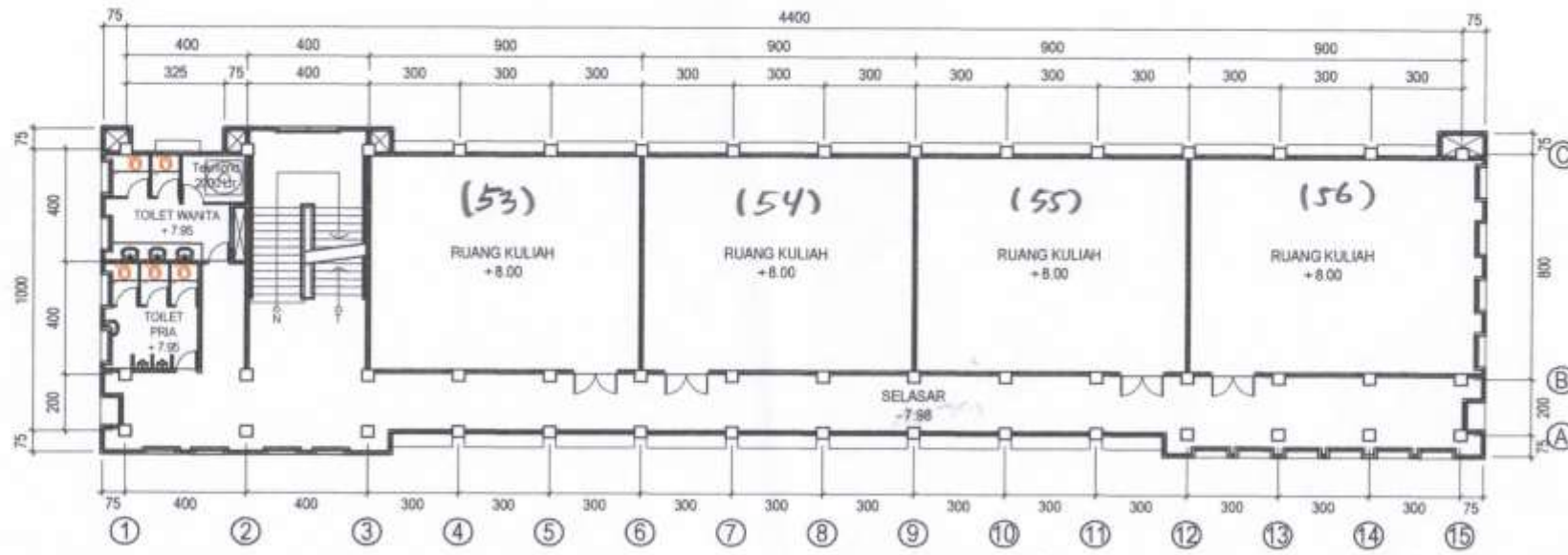
DENAH LANTAI - 3 GD. KULIAH FISIP C SKALA 1 : 175
